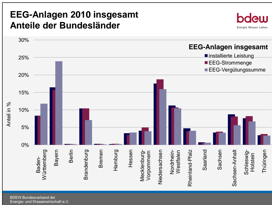
Abb. 28: EEG-Gesamt: Regionale Verteilung von Leistung, Strommengen und Vergütung
