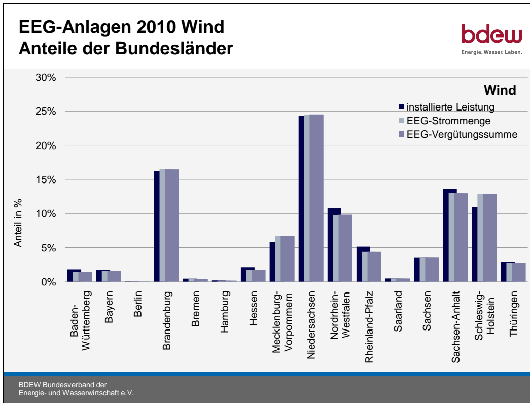
Abb. 29: Windenergie: Regionale Verteilung von Leistung, Strommengen und Vergütung
