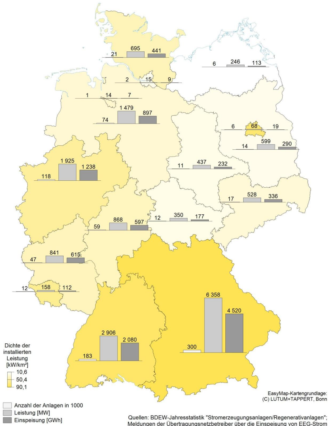
Abb. 9: Nutzung der Photovoltaik 2010
