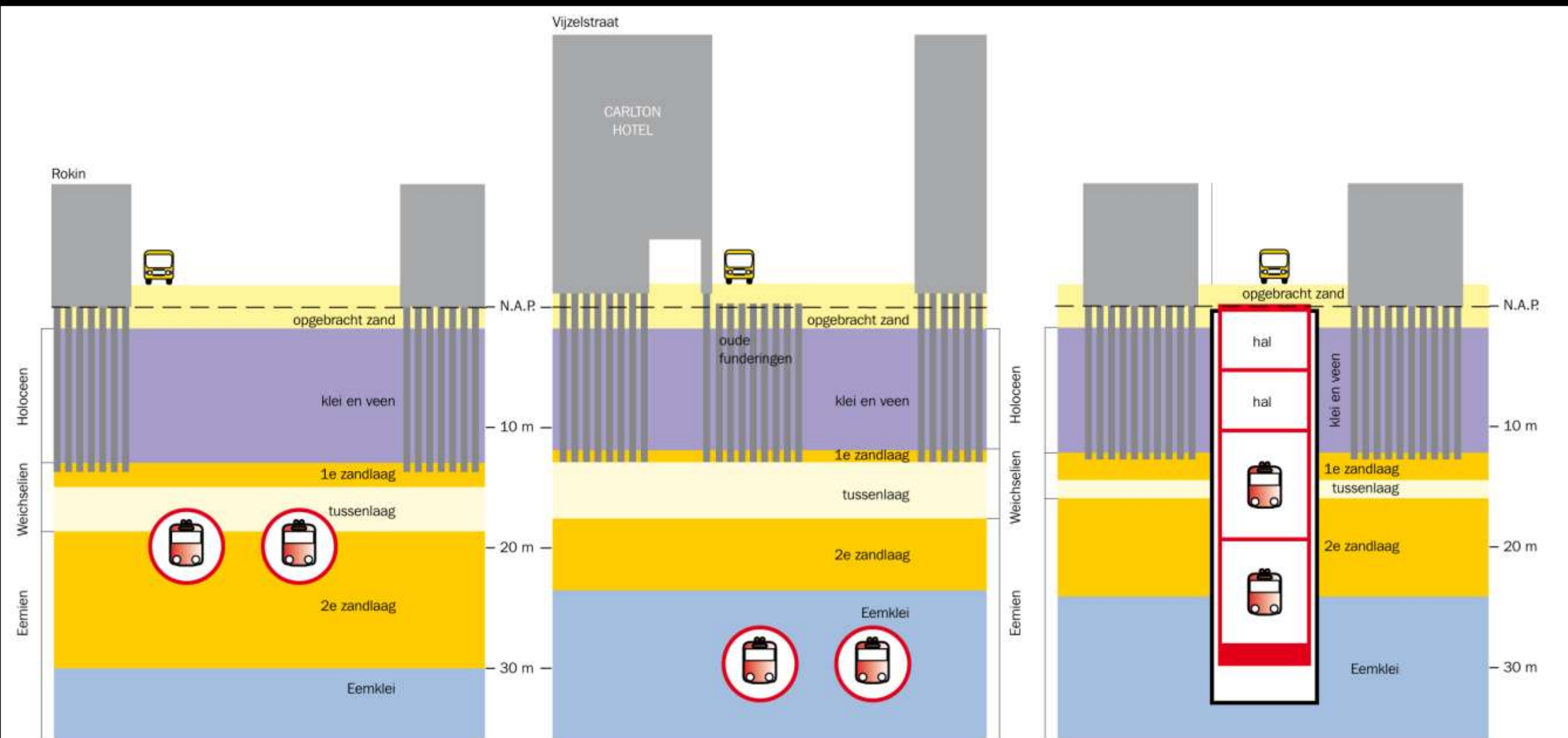
De ligging van de metrobuizen onder het Rokin en de Vijzelstraat.
