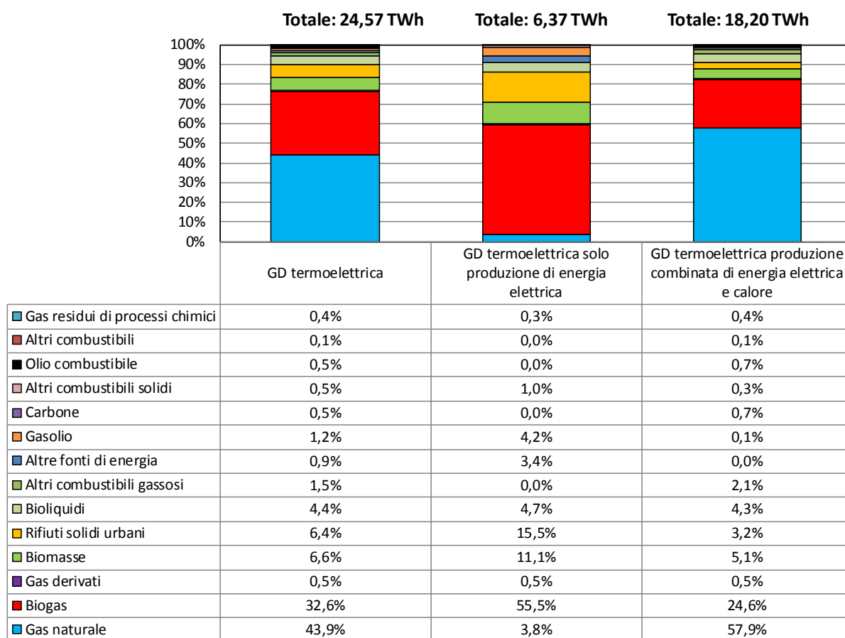
Figura 7 4 : Produzione di energia elettrica dalle diverse fonti utilizzate nell'ambito della GD da termoelettrico
