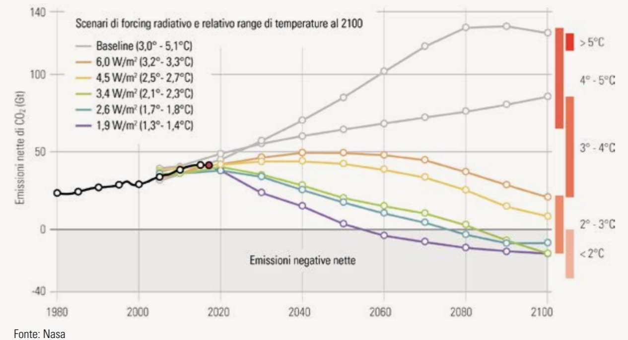
Figura 3 Scenari al 2100 per emissioni di gas serra e aumenti delle temperature globali
