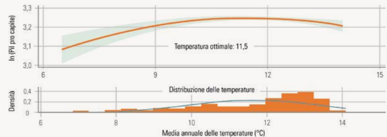
Figura 13 Relazione stimata tra Pil pro capite e temperatura in Italia
