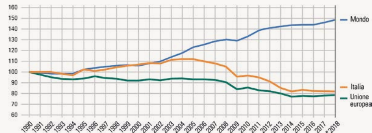
Figura 21 Andamento delle emissioni di gas serra nel mondo, nella Ue28 e in Italia, 1990-2018 (valori indice 1990=100), *dati provvisori
