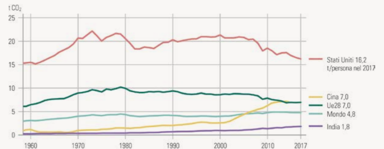
Figura 57 Emissioni pro capite dei principali emettitori (tCO 2 )
