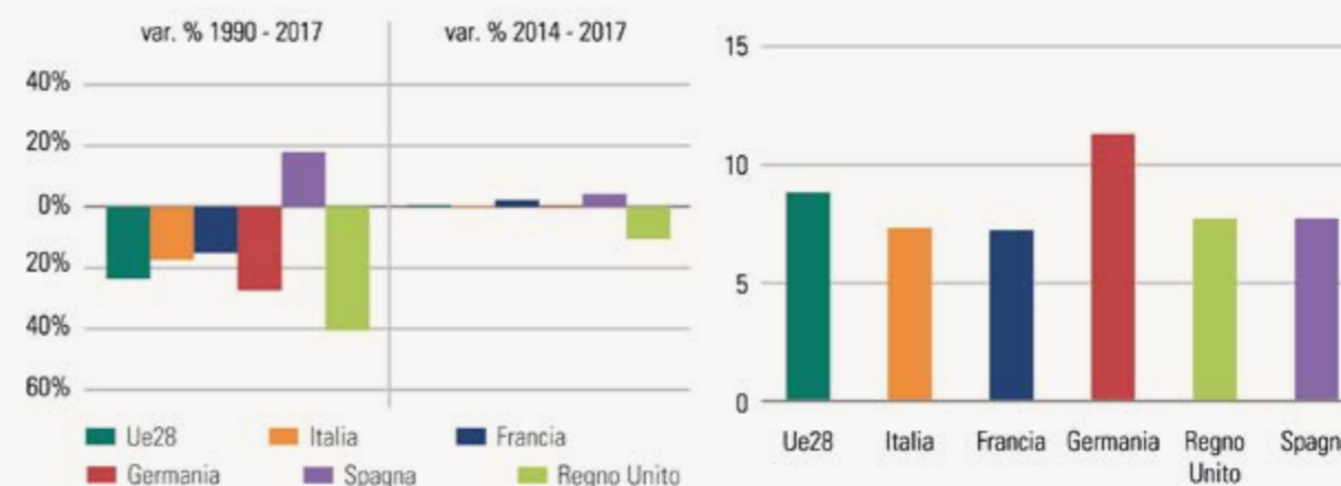
Figura 20 Andamento delle emissioni di gas serra nelle principali economie europee: variazioni percentuali (%), a sx) ed emissioni pro capite (tCO 2 eq), a dx)
