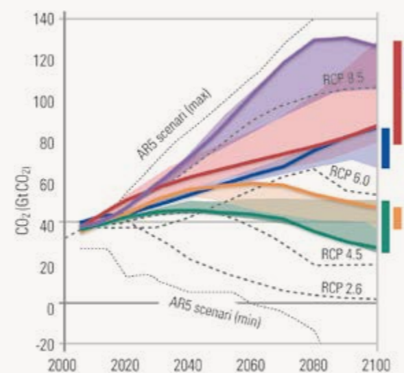
Figura 7 Emissioni future di CO 2 per i diversi Ssp
